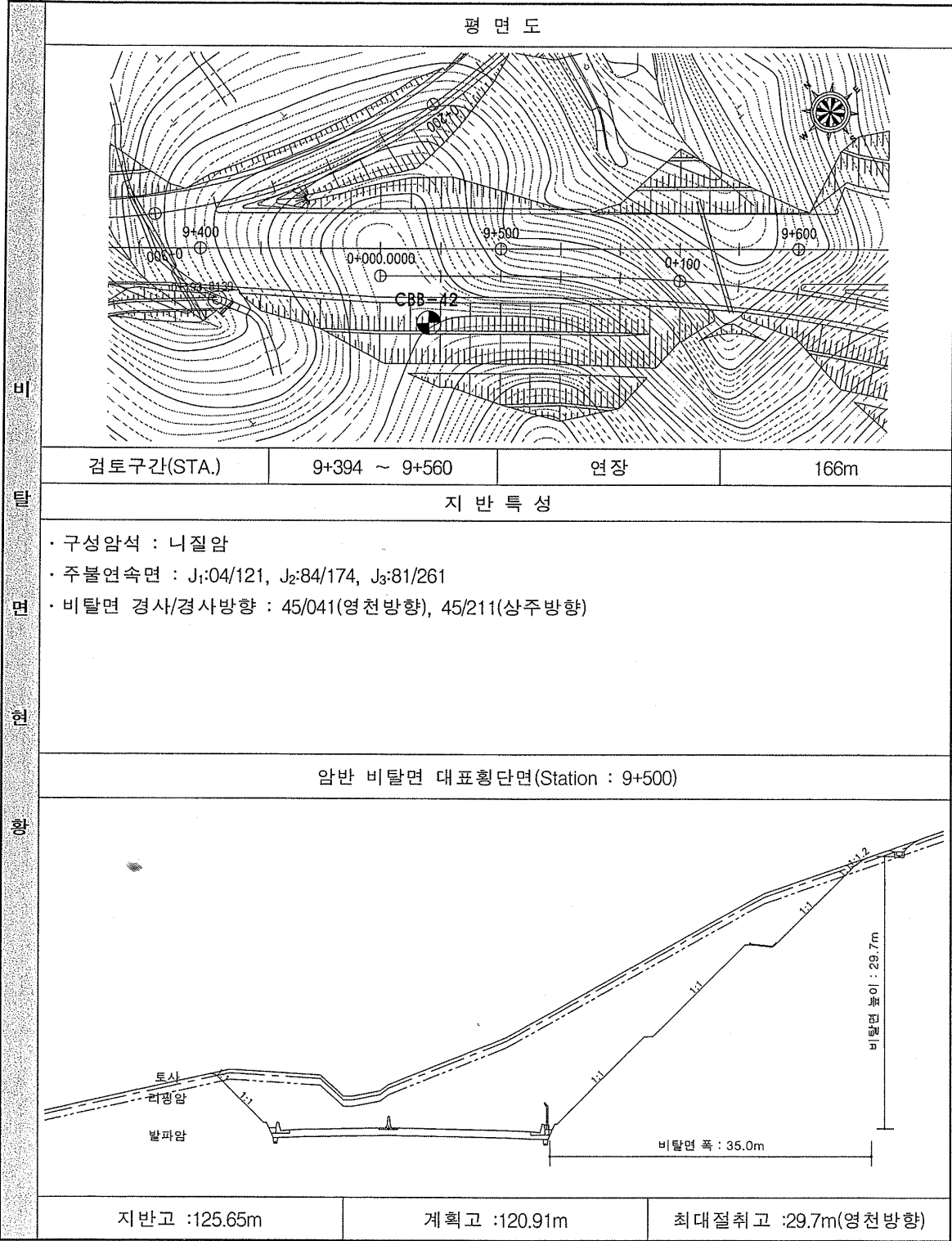
(16) 깎기 22구간
