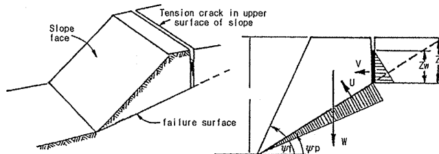
< 비탈면 정상부쪽에 인장균열이 있는 비탈면 >
