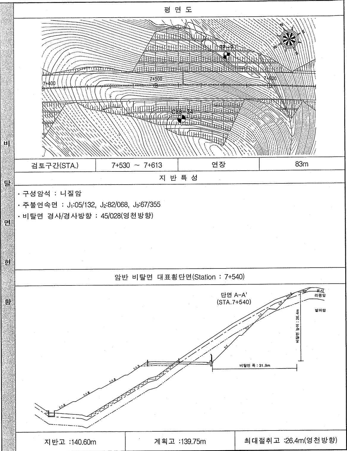
(11) 깎기 17구간
