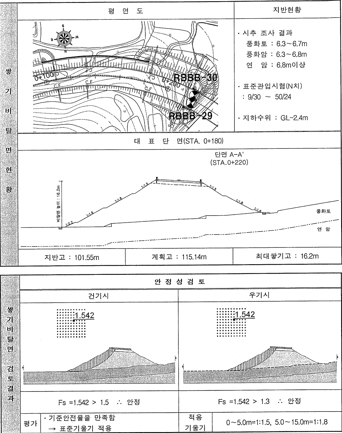
(4) 화산 JCT RAMP-A (STA. 0+000~1+723, L= 1,723m)
