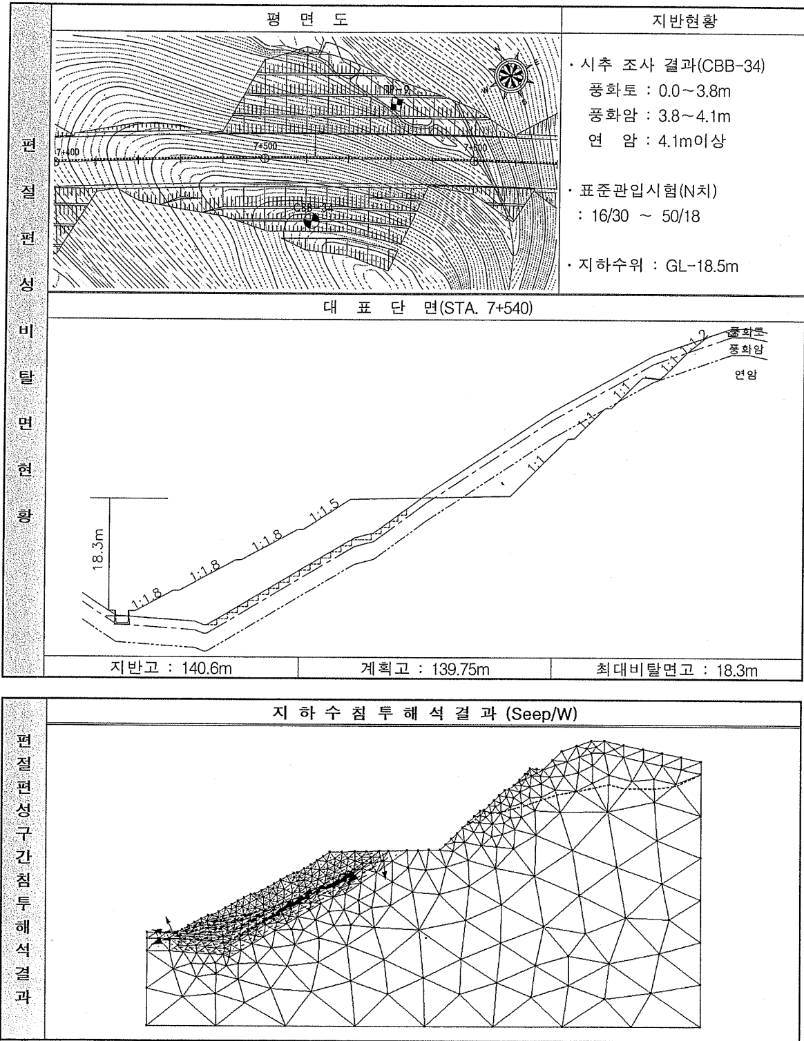
(5) 편절편성구간 (STA. 7+480~7+620, L= 140m)
