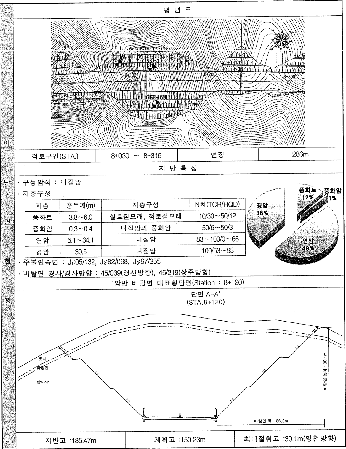
(13) 짝기 19구간
