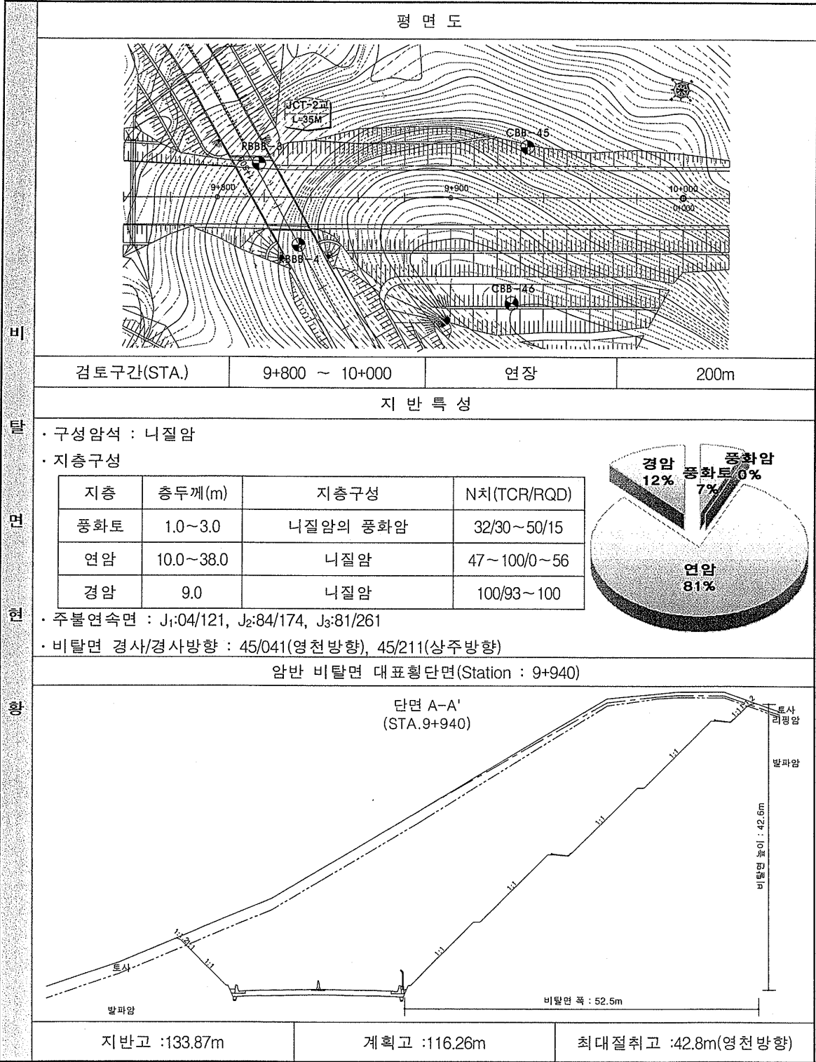
(18) 깎기 24구간
