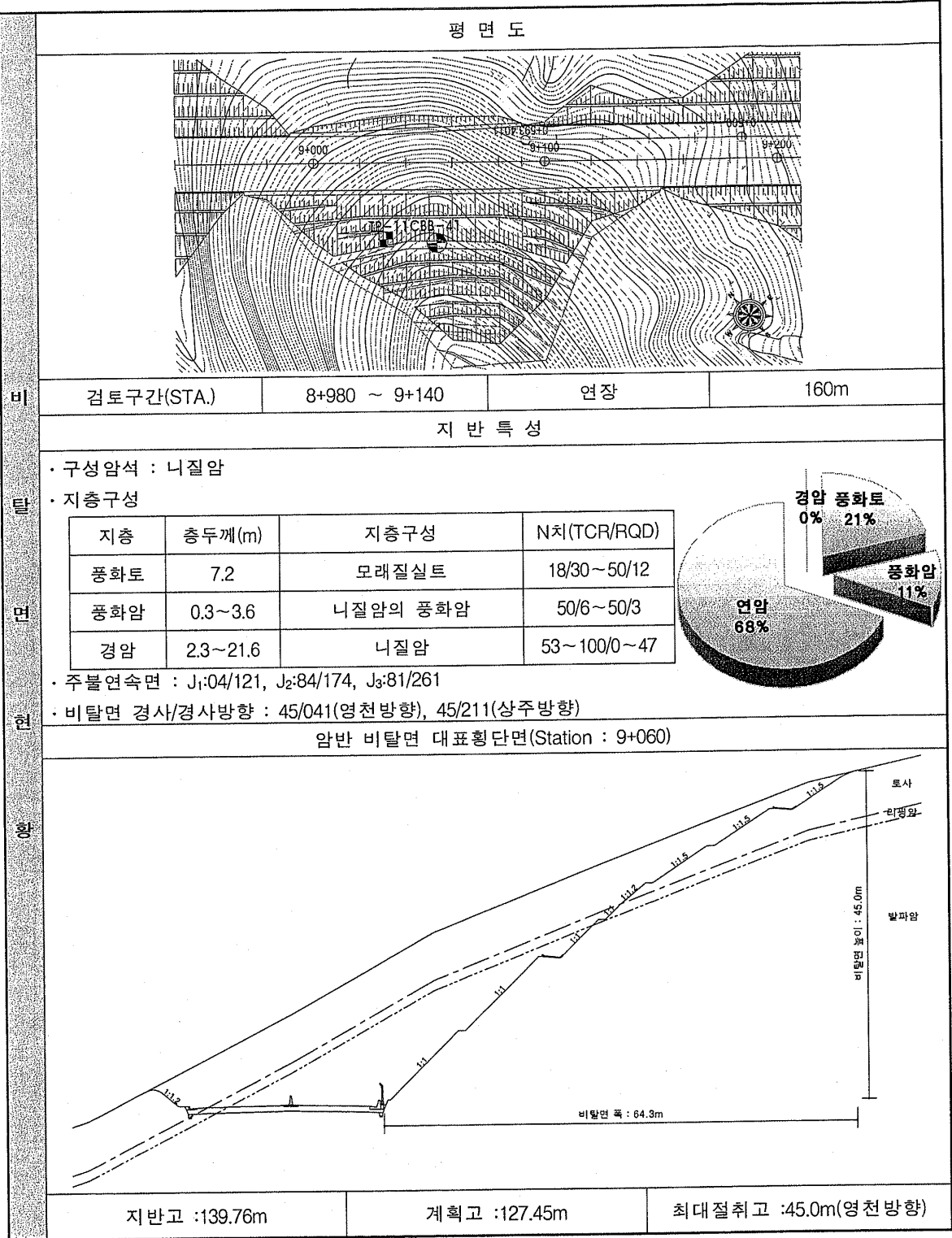
(15) 깎기 21구간
