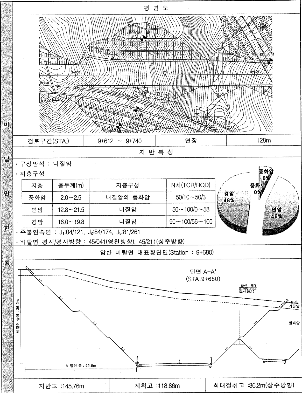
(17) 깎기 23구간
